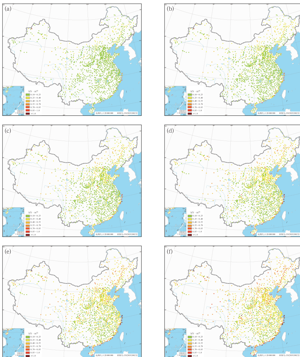
图 1 不同重现期的全国基本风压分布
