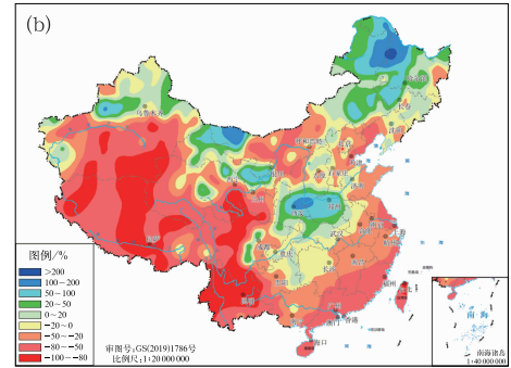
图 3 (a)1961/1962—2025/2026 年冬季全国平均降水量变化及(b)2025/2026 年冬季全国降水量距平百分率空间分布
