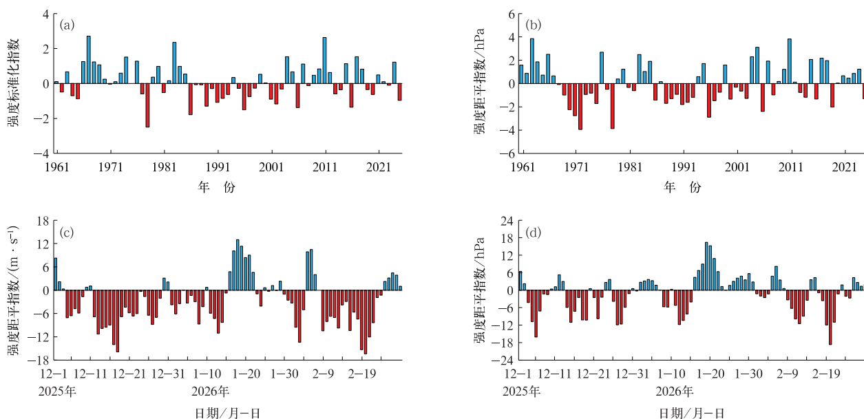
图 7 (a,b)1961/1962—2025/2026 年冬季(a)强度标准化指数和(b)强度距平指数历年变化,(c,d)2025/2026 年冬季强度距平指数逐日演变 (a,c)东亚冬季风,(b,d)西伯利亚高压
