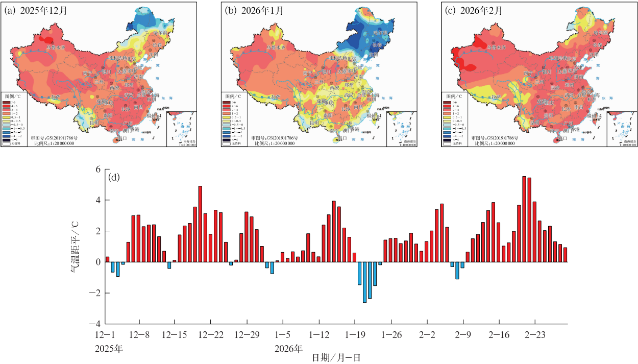
图 2 2025/2026 年冬季全国(a~c)逐月平均气温距平分布和(d)平均气温距平逐日演变
