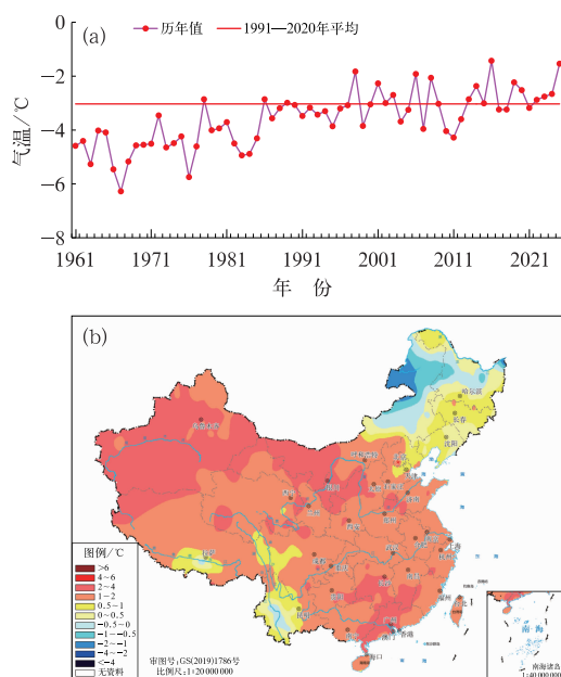
图 1 (a)1961/1962—2025/2026 年冬季全国平均气温历年变化及(b)2025/2026 年冬季全国平均气温距平空间分布
