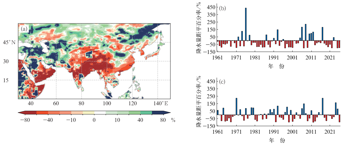
图9 (a)2025/2026 年冬季亚洲地区降水量距平百分率空间分布及(b,c)1961/1962—2025/2026 年冬季我国(b)南疆地区和(c)内蒙古中西部降水量距平百分率历年变化
