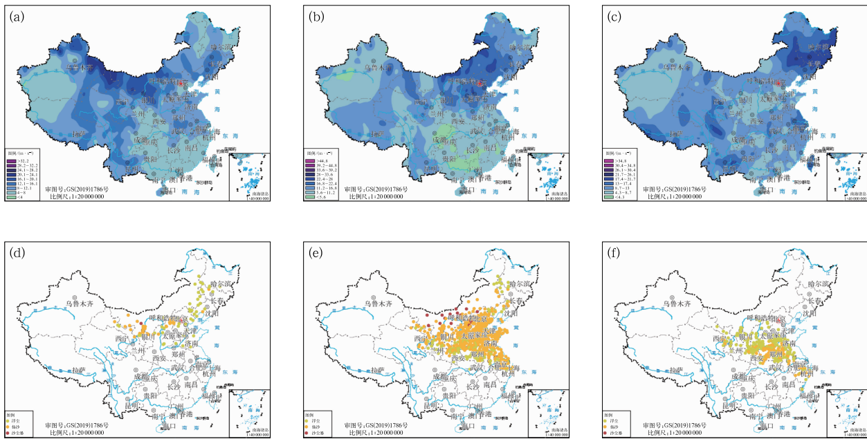
图 13 2026 年 2 月 (a, d)20 日, (b, e)21—22 日及 (c, f) 23 日的全国 (a~c)地面风速及 (d~f)沙尘过程强度分布
