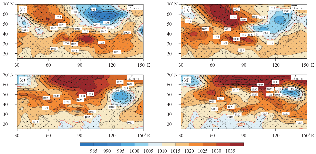
图 12 2026 年 2 月 (a)19 日, (b)20 日, (c)21—22 日及 (d)23 日海平面气压 (等值线和填色, 单位: hPa) 和 850 hPa 风场距平 (风矢)
