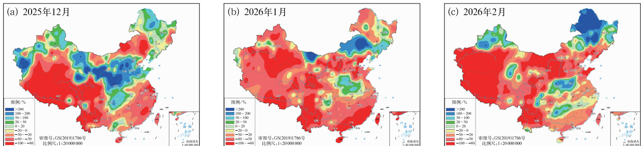
图 4 2025/2026 年冬季全国逐月平均降水量距平百分率分布
