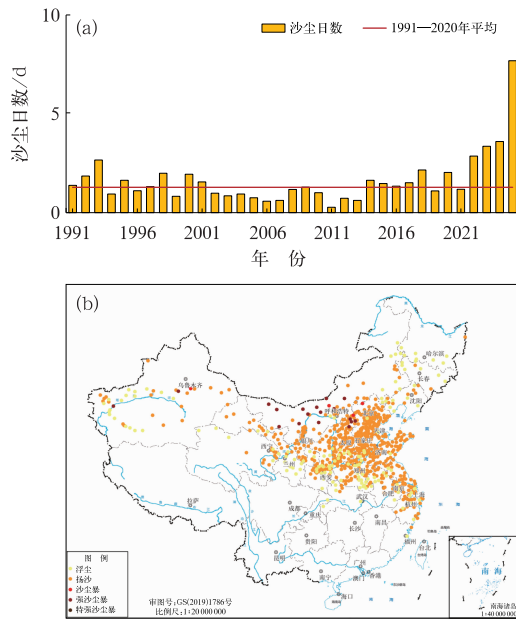
图8 (a)1961/1962—2025/2026 年冬季沙尘日数历年变化及(b)2026 年 2 月 20—23 日全国沙尘过程强度分布
