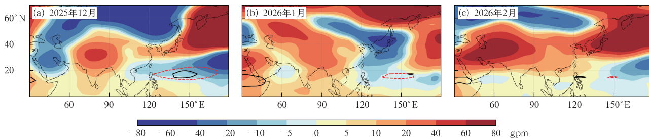
图 6 2025/2026 年冬季逐月 500 hPa 位势高度距平场 Fig. 6 Monthly geopotential height anomaly at 500 hPa in the 2025/2026 winter
